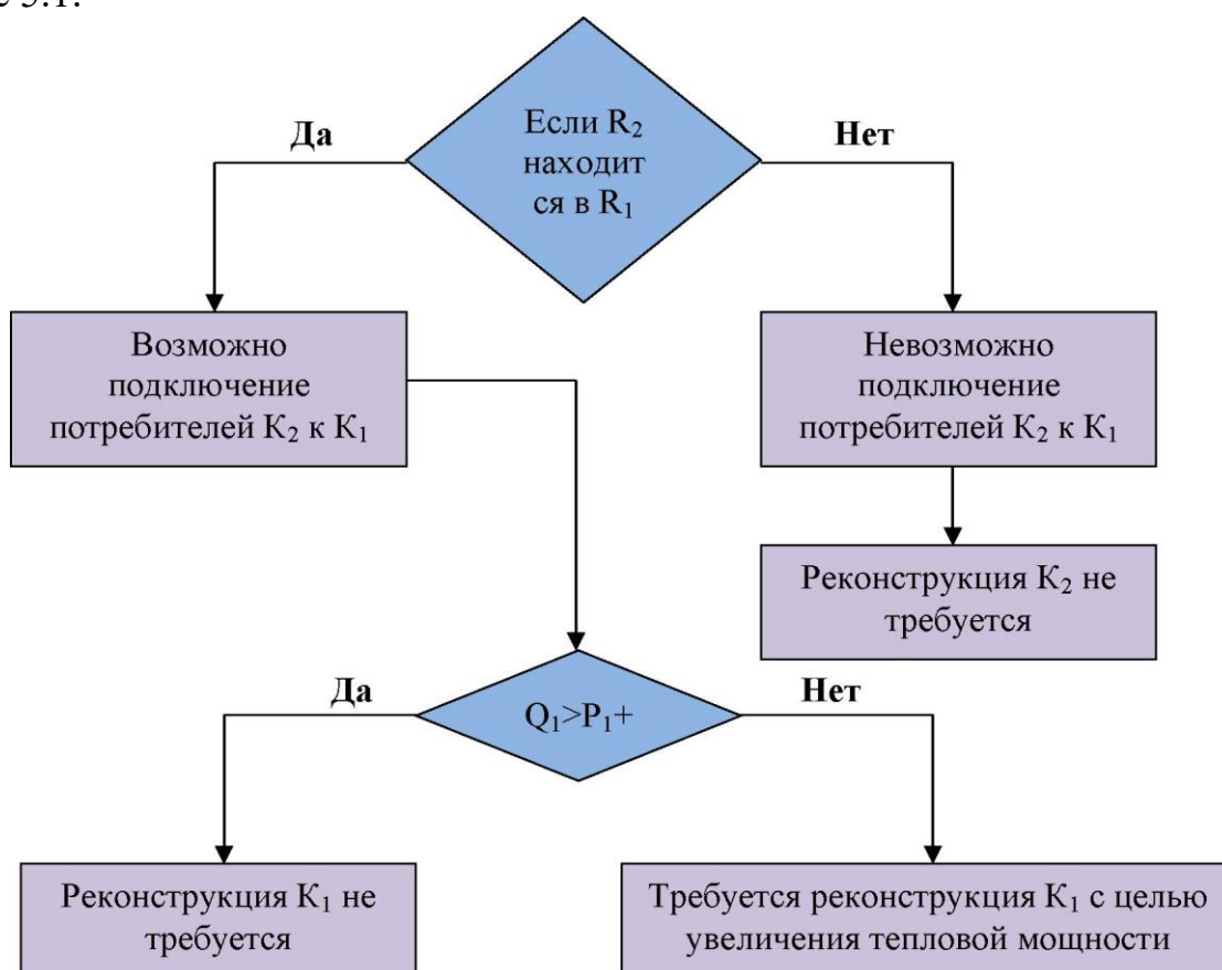
Рисунок 5.1 - Блок-схема обоснования реконструкции котельной K_2 , K_2 - котельная №1 и котельная №2; R_1 , R_2 - радиусы эффективного теплоснабжения котельной №1 и котельной №2; Q_1 - тепловая мощность котельной №1; P_1 , P_2 - подключённая тепловая нагрузка к котельной №1 и котельной №2.
